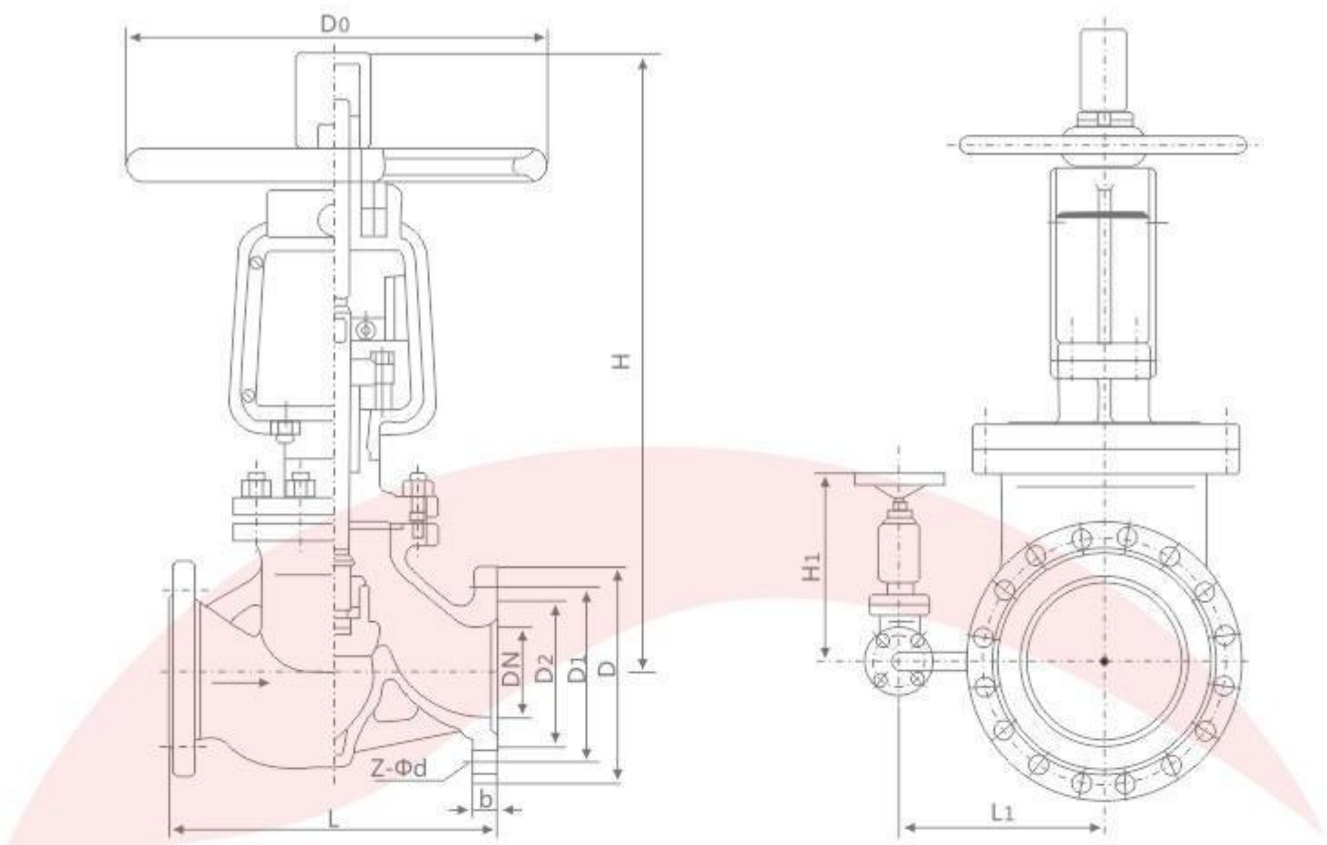
主要外形及和连接尺寸 Main external and connection dimension JB/T79.1 单位Unit:mm
